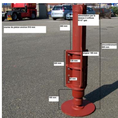
STABILISATEUR HYDRAULIQUE C 510 HPB - SAV UNIQ 234-012
