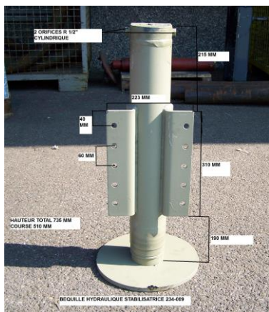
STABILISATEUR HYDRAULIQUE C 510 NEUMEISTER 234-009
