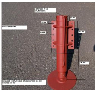
STABILISATEUR HYDRAULIQUE ARRIERE DE 90/70 C 350 234-010
